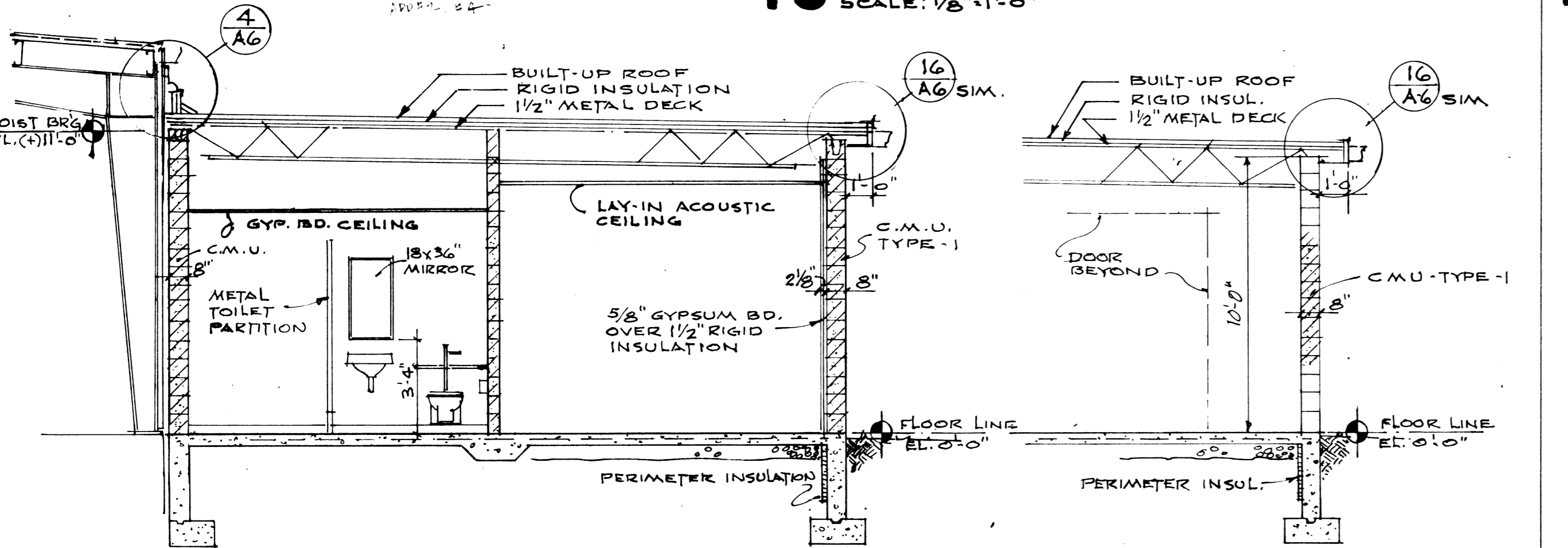
18 SECTION SCALE: 1/4" = 1'-0"
