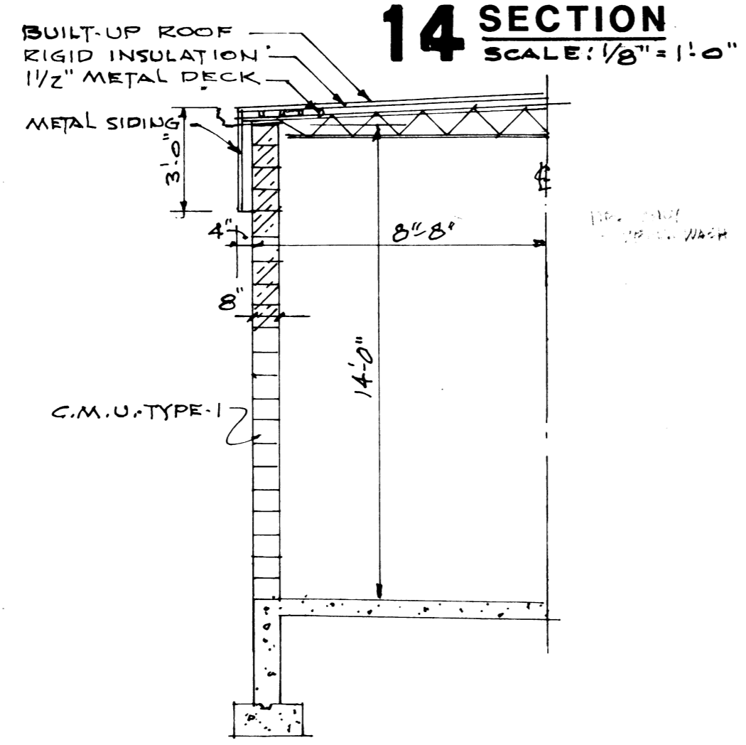
14 SECTION SCALE: 1/8" = 1'-0"
