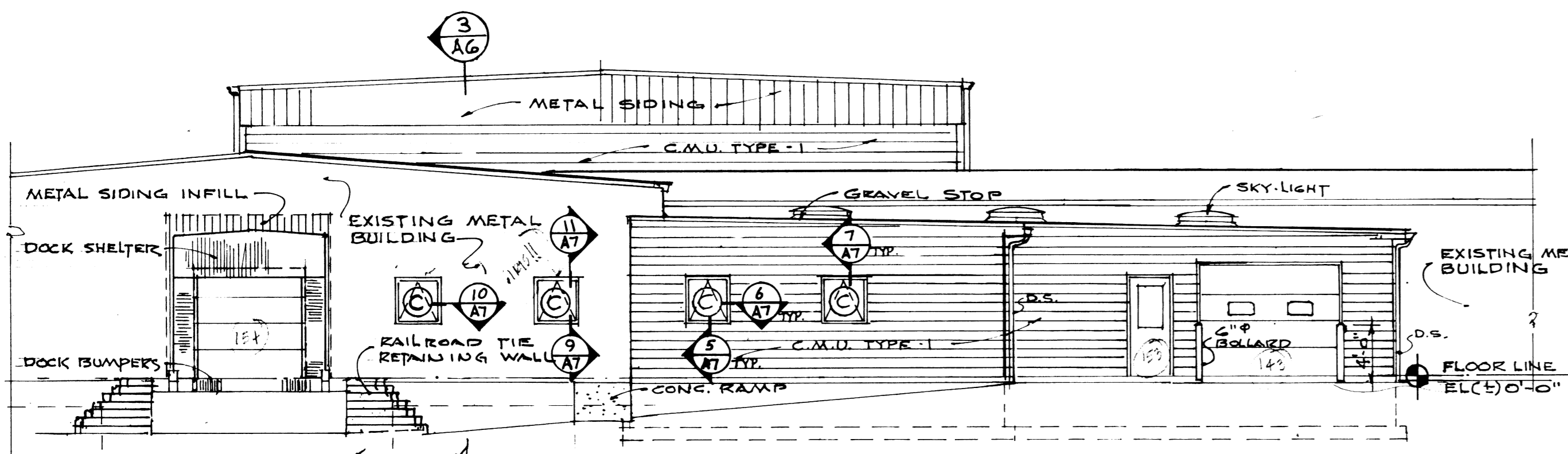
15 SOUTH ELEVATION SCALE: 1/8" = 1'-0"
