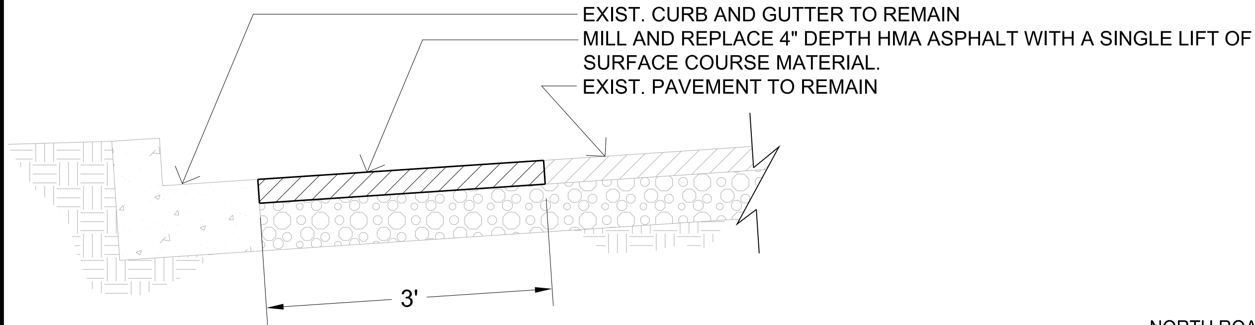
2 LEFT STA 25+00 TO STA. 48+64 4 NOT TO SCALE
