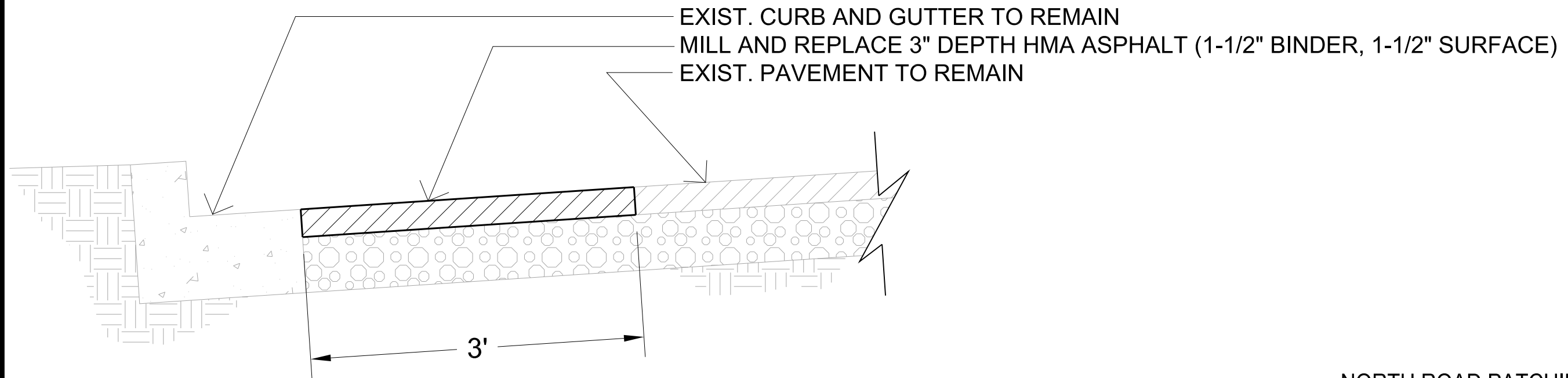
2 LEFT STA 5+41 TO STA. 25+00 4 NOT TO SCALE
