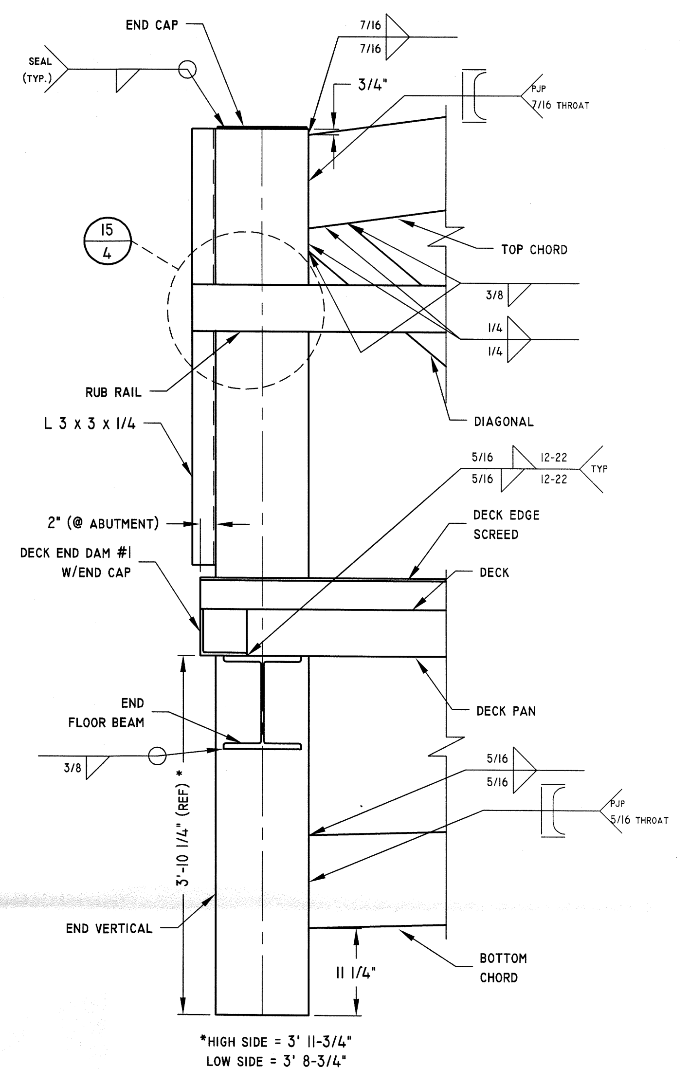
13 SECTION A-A SCALE: 1" = 1' 0"
