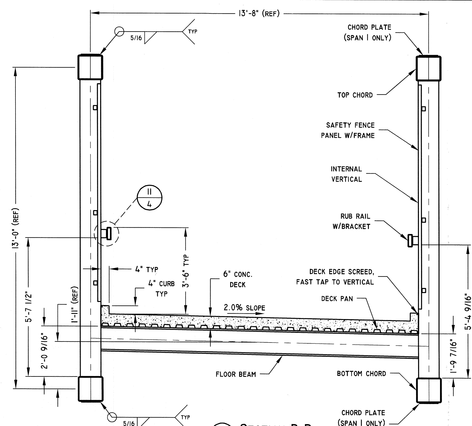
9 SECTION B-B SCALE: 1/2" = 1' 0"
