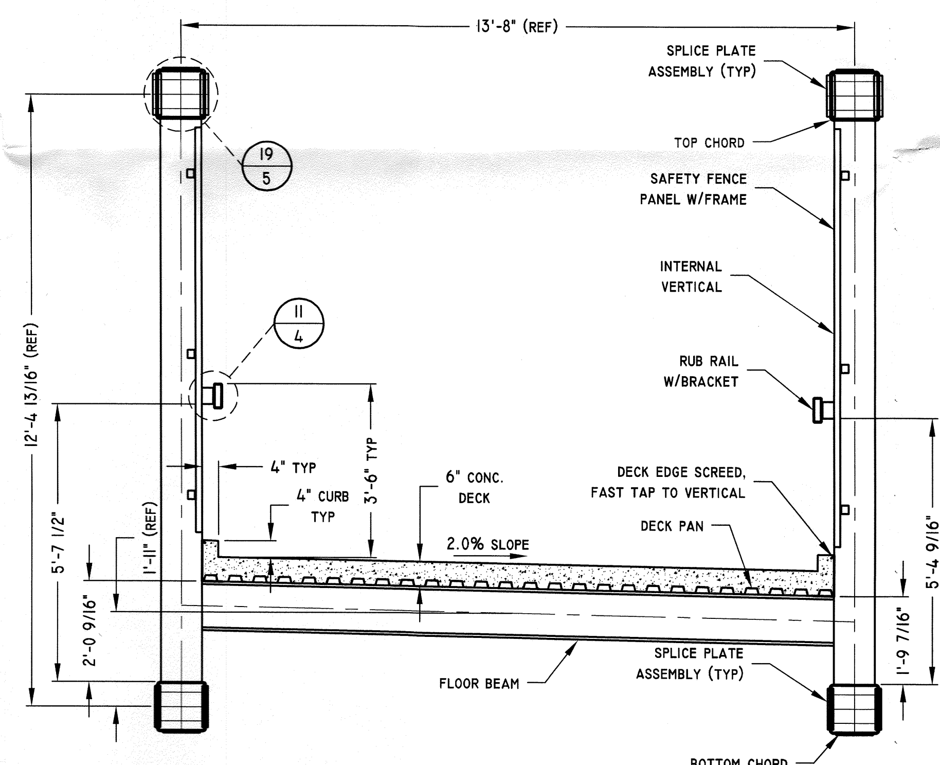
12 SECTION C-C SCALE: 1/2" = 1' 0"
