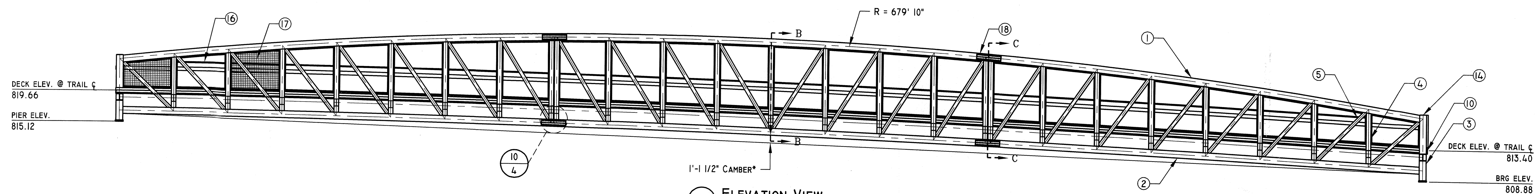
5 ELEVATION VIEW SCALE: 1/8" = 1' 0"
