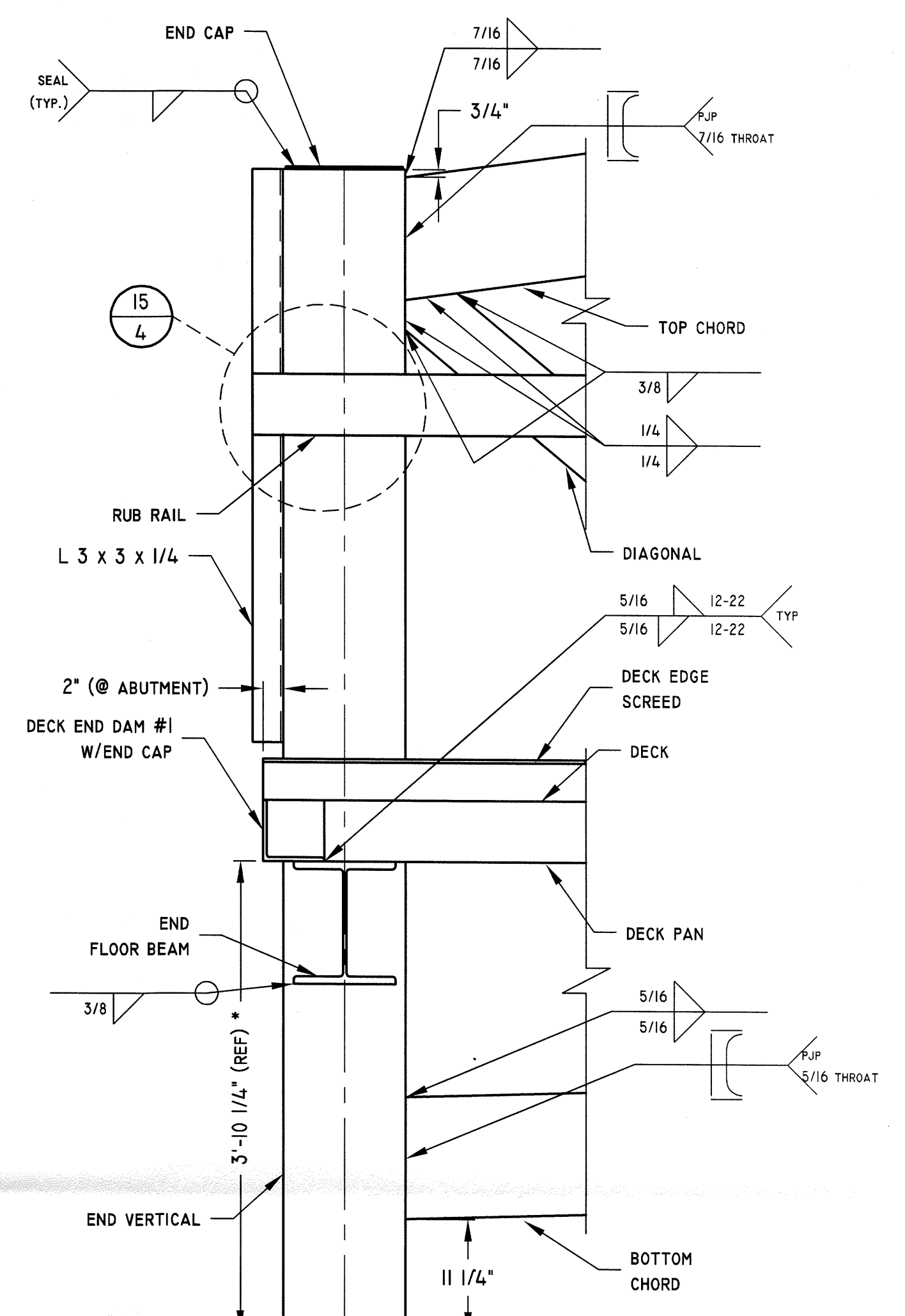
13 SECTION A-A SCALE: 1" = 1' 0"
