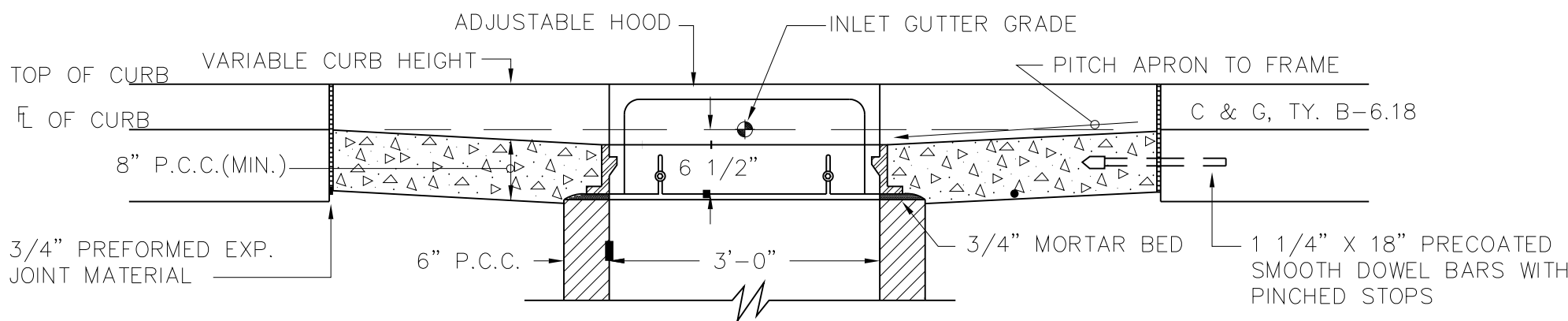
SECTION A-A
